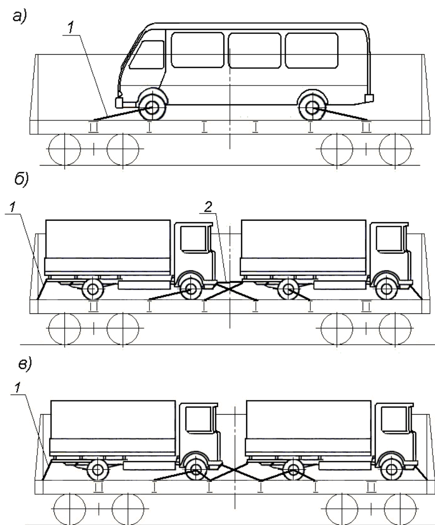
Рисунок 18 – Размещение и крепление техники на обрешиненных колесах в полувагоне 1 – растяжка; 2 – увязка
