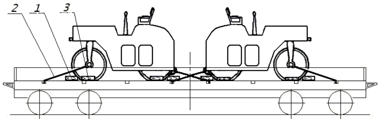
Рисунок 15 – Размещение и крепление техники на металлических колесах без гребней на платформе
